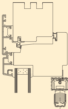
Einbausituation Glaslichte
